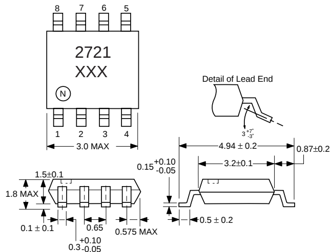
UPC2721GV/UPC2722GV PACKAGE OUTLINE S08
