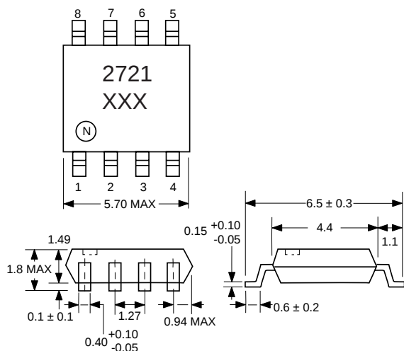
UPC2721GR/UPC2722GR PACKAGE OUTLINE G08
